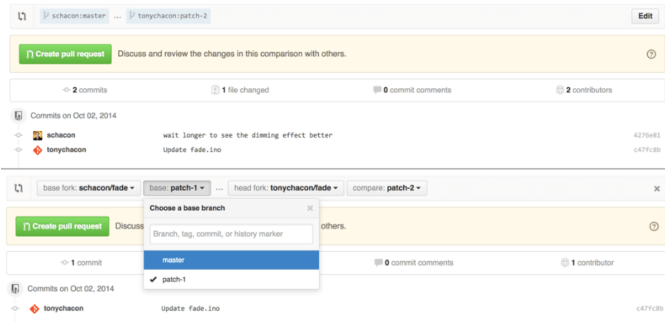
Figure 118. Cambio manual de la rama o del fork en un pull request.
