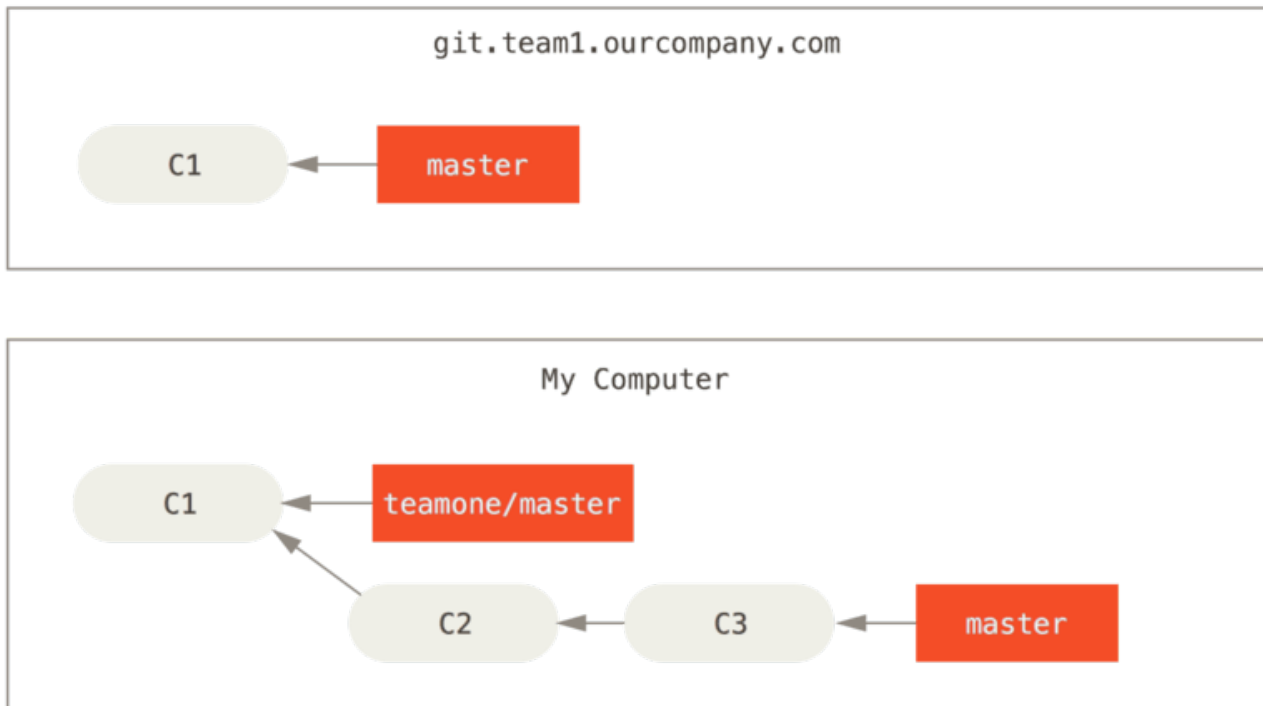
Figure 44. Clonar un repositorio y trabajar sobre él
